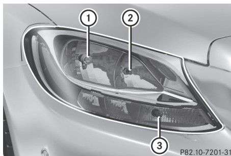
Projecteur halogène
