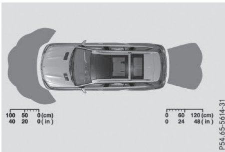
Capteurs avant
