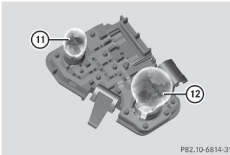
Porte-ampoule
