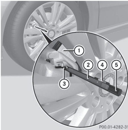
Roue avant
